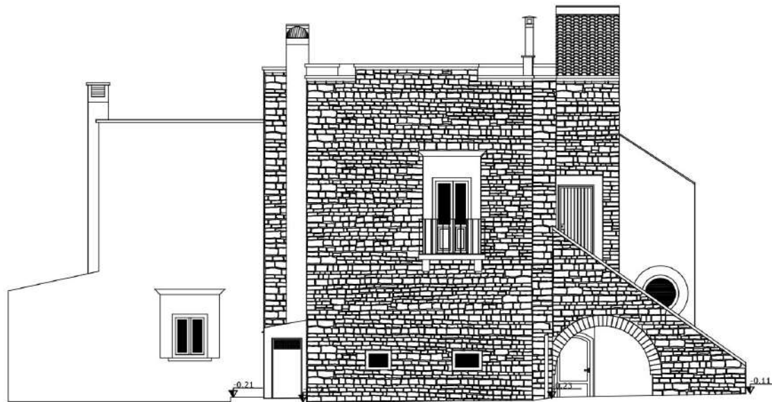
PROSPETTO SUD
