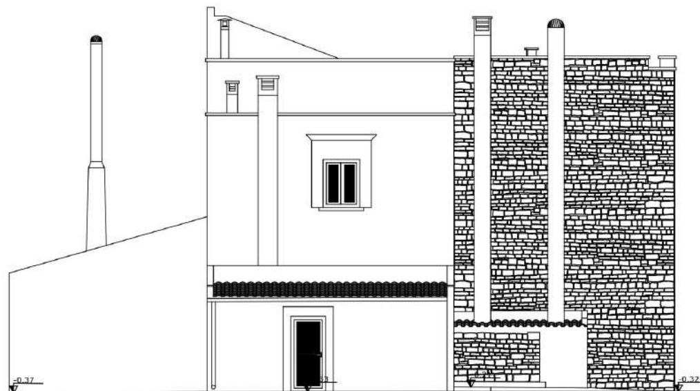
PROSPETTO OVEST
