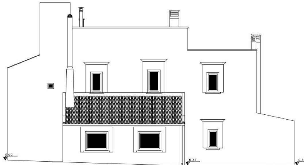
PROSPETTO NORD
