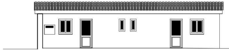
PROSPETTO OVEST
