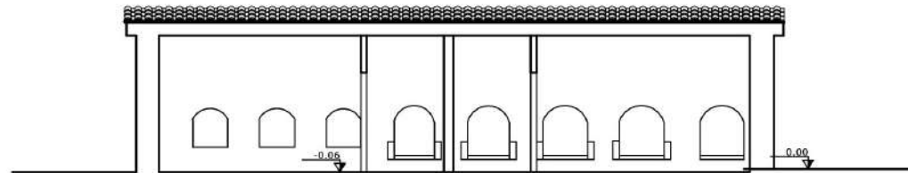
SEZIONE B-B
