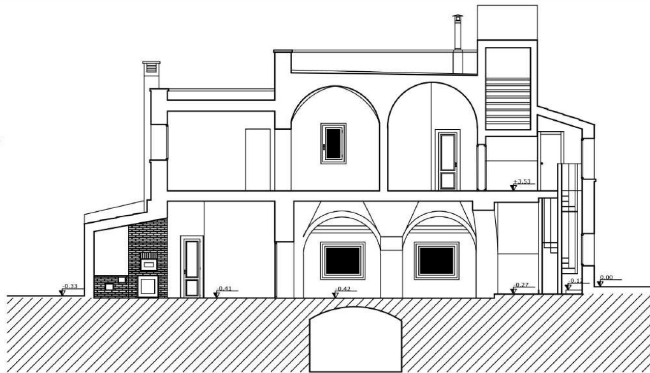
SEZIONE A-A
